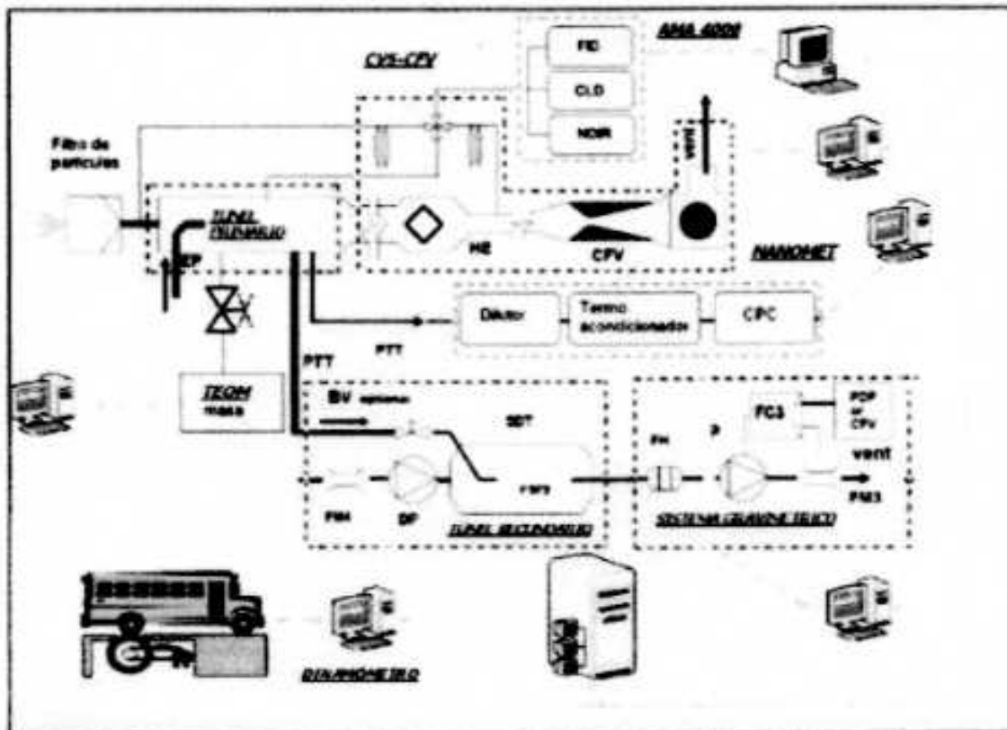
Figura Nº4. Esquema general de un laboratorio de vehículos pesados
